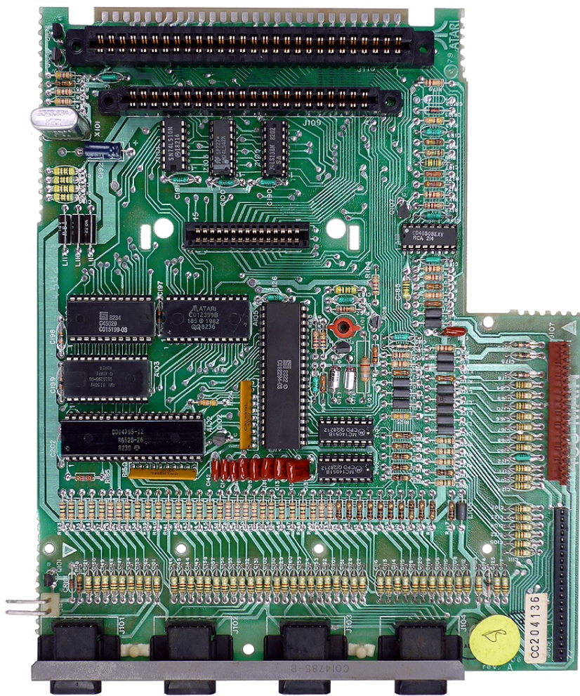
Abb. 4.7: Foto Mainboard 400
