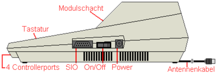
Abb. 4.1: Anschlüsse 400
