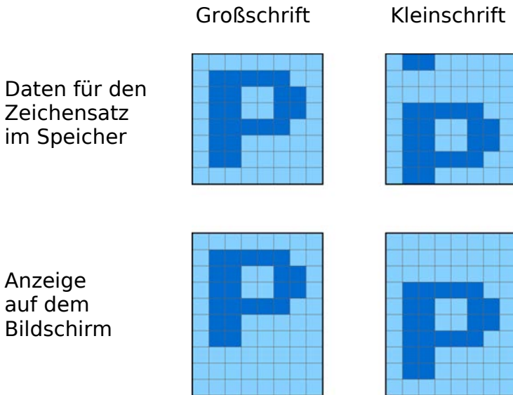
Abb. 2.1: Beispiel für die Anwendung des ANTIC-Modus 3
