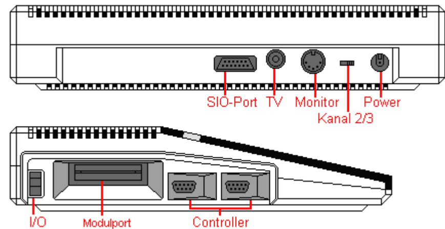
Abb. 4.19: Anschlüsse 1200XL (NTSC)
