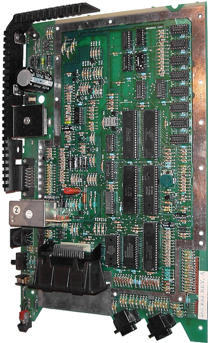
Abb. 4.22: Foto Mainboard 1200XL (NTSC)
